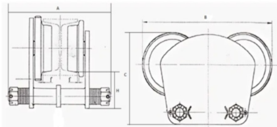
Рисунок 2. Холостая ходовая тележка.
