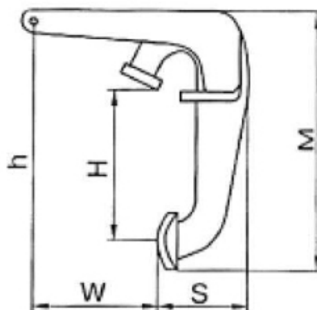
Рисунок 1 Размеры захвата.
