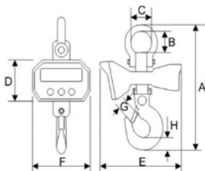
Рисунок 1. Технические характеристики весов.
