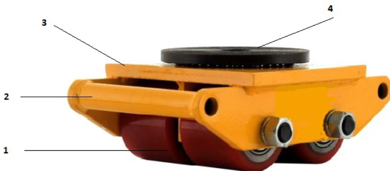
Рисунок 1. Устройство тележки
