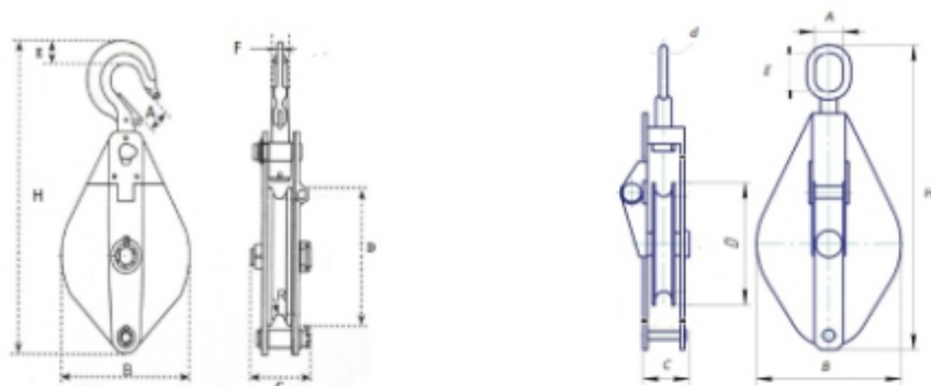
Рисунок 1. Размер блоков
