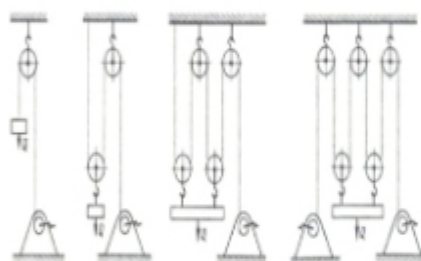
Рисунок 2. Применение блоков
