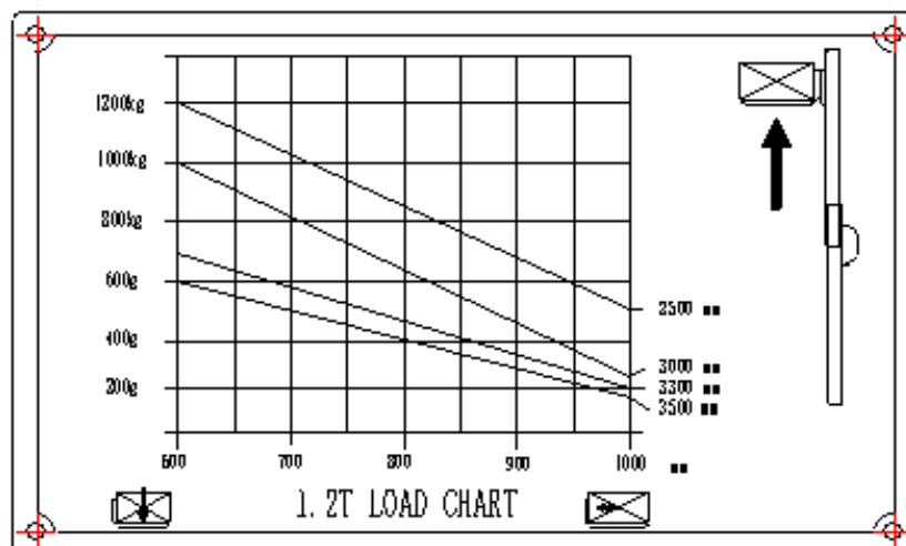
Рис. 4 - График грузоподъемности для CDD12RDS-E
