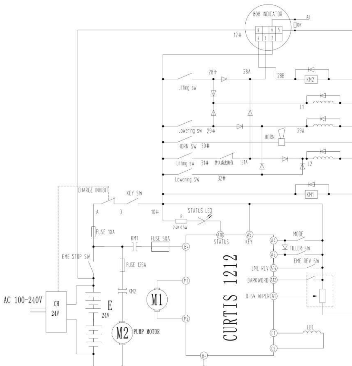
Схема 2. Принципиальная электрическая схема
