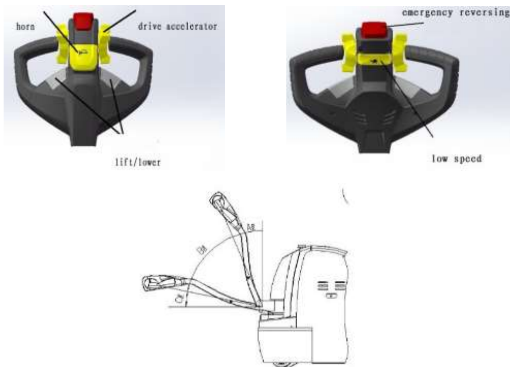
Рис.5 Horn – звуковой сигнал; lift/lower – кнопки управления «вверх»/«вниз»; drive accelerator – высокая скорость; emergency reversing – кнопка аварийного обратного движения; low speed – медленная скорость.
