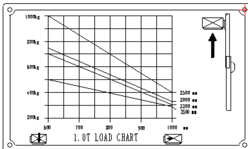
Рис. 3 - График грузоподъемности для CDD10RDS-E
