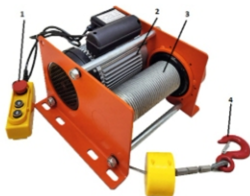
Рисунок 1. Конструкция лебедки
